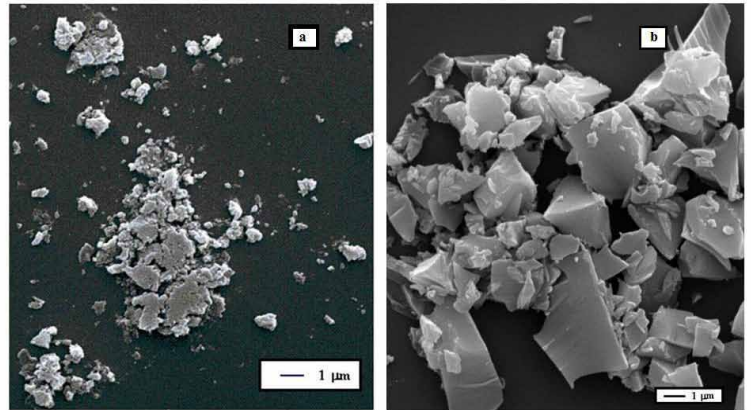
Figura 5. Imágenes de microscopía electrónica de barrido (SEM) de los medicamentos homeopáticos (a) Pulsatilla 1CH y (b) Pulsatilla 2CH, en donde la sustancia de partida tiene la mayor probabilidad de encontrarse presente. Los materiales observados son conglomerados de nanopartículas tal y como se han formado en el área capturada en la imagen. Una gota de muestra fue secada en un cubreobjetos de vidrio bajo flujo de aire laminar limpio y el nanomaterial fue buscado en esa gota en una vasta área a nanoescala. Siempre que se encontraron materiales con alguna forma interesante, la correspondiente área extremadamente pequeña fue capturada en imagen.
