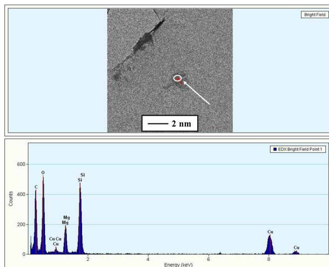
Figura 10. Análisis de energía dispersiva de rayos X (EDX) del área seleccionada utilizando rejilla de cobre revestida con carbono para el medicamento homeopático Colchicum 15CH que muestra un alto contenido de silicio.
