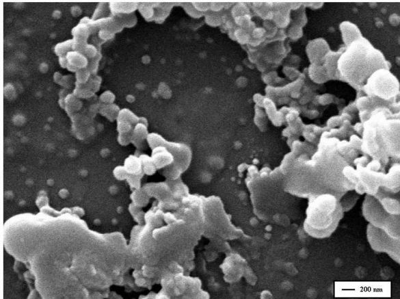
Figura 3. Imagen de microscopía electrónica de barrido (SEM) de agua 14CH (agua pura usada como material de partida) que muestra nanomateriales.
