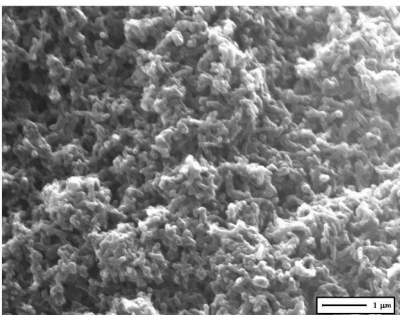
Figura 4. Imagen de microscopía electrónica de barrido (SEM) de Colchicum 15CH: un control preparado en frascos de plástico que muestra nanomaterial. Sin embargo, su apariencia difiere de las muestras preparadas en recipientes de vidrio.
